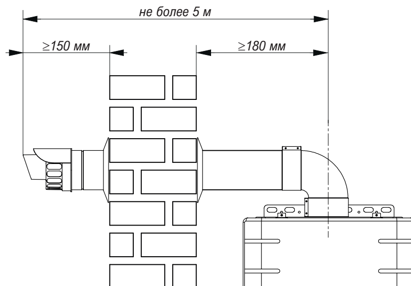
Рисунок 10. Коаксиальный дымоход.
